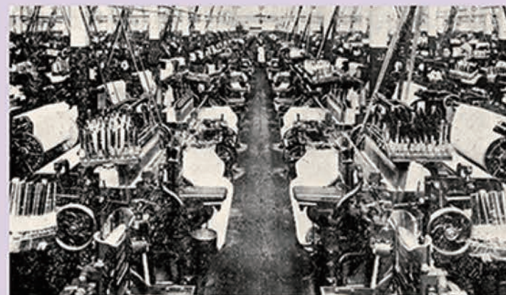
豊田紡織刈谷工場におけるG型自動織機 Toyoda Automatic Loom, Type G at Toyoda Boshoku Kariya Plant
